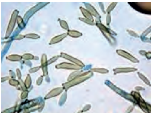
Abb.10: Cladosporium
