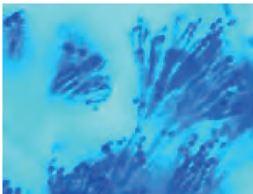
Abbildung 13: Penicillium
