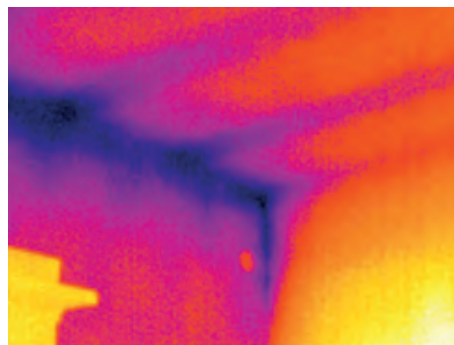
Abb. 5: Diese Infrarot-Aufnahme zeigt eine typische materialbedingte Wärmebrücke. Deutlich zeichnet sich in der Farbe Blau der betonierete Deckenrost so wie die Stahlbeton-Deckenträger ab.
