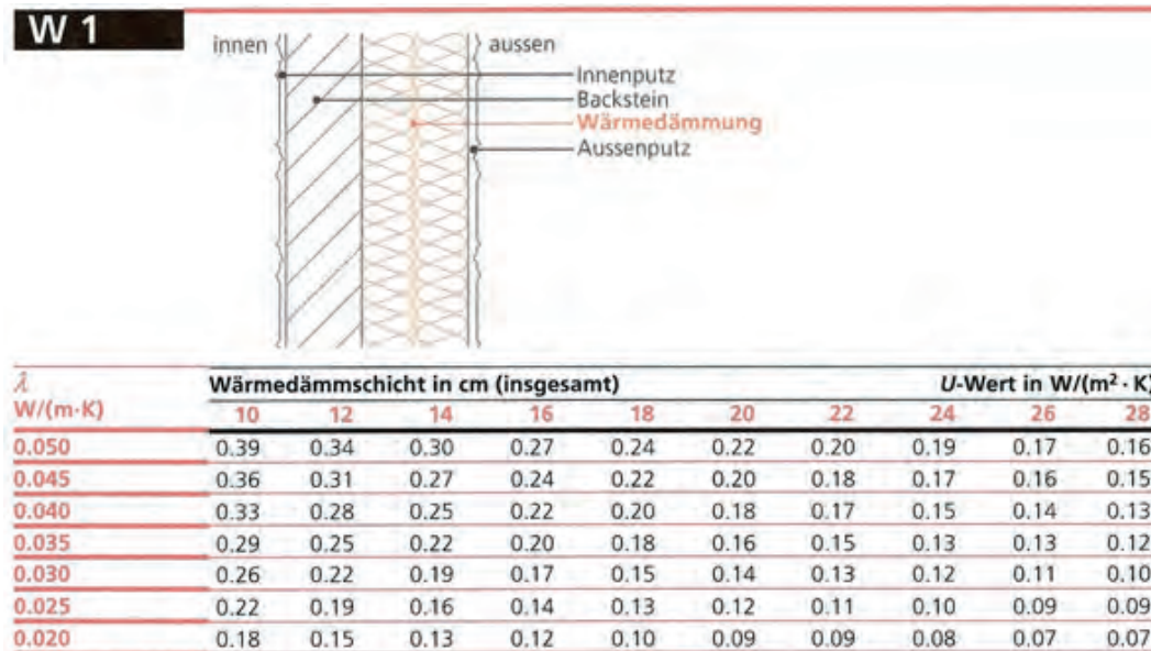
Abbildung 4: Wärmedämmschichten
